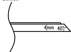
横断面
