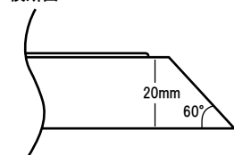
横断面
