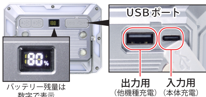
ライト本体の充電接続参考図
