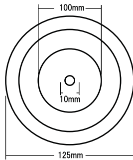
取り付け面寸法 (M-125)
