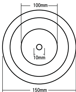
取り付け面寸法 (M-150)
