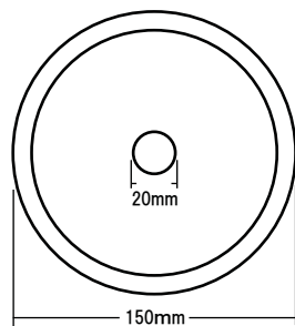
取り付け面寸法 (D-150)
