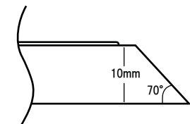
横断面
