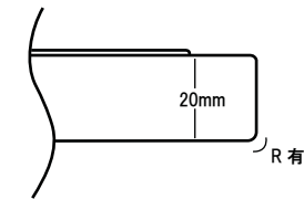
横断面
