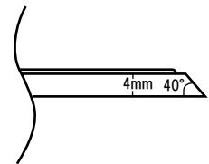
横断面
