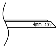
横断面
