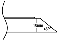
横断面
