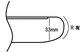
横断面
